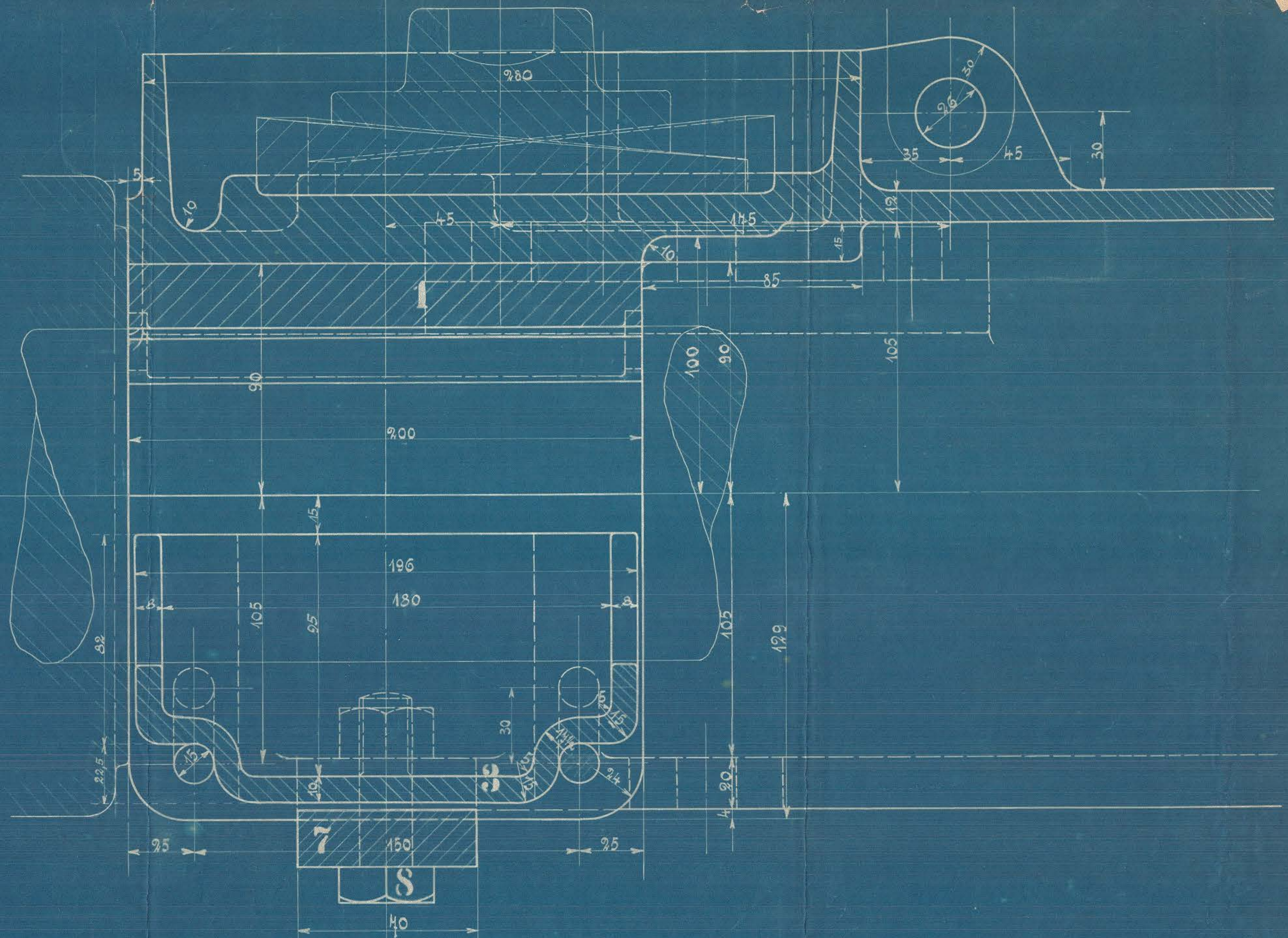
Schnitt A-B
